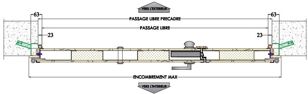
Joint d'étanchéité enfoncé sur le cadre
