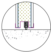
Plinthe coupe vent automatique (selon modèle)
